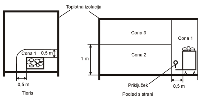
Slika 10: Mere con v savni (SIST HD 60364-7-703: 2005)
