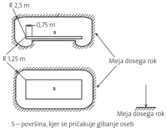
Slika 6: Postavitev zunaj dosega rok (vir: SIST HD 60364-4-41: 2007, slika B1)
