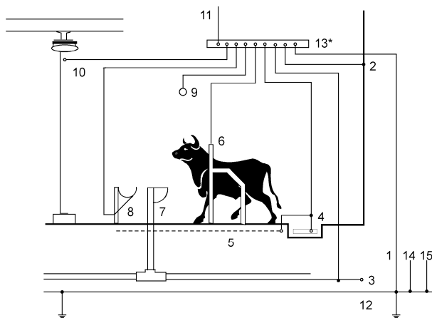
Slika 11: Izvedba zaščite z izenačitvijo potenciala v hlevu
