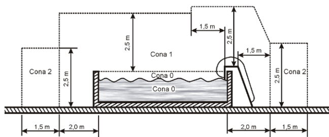
Slika 9: Mere con za plavalne bazene nad zemeljskim nivojem
